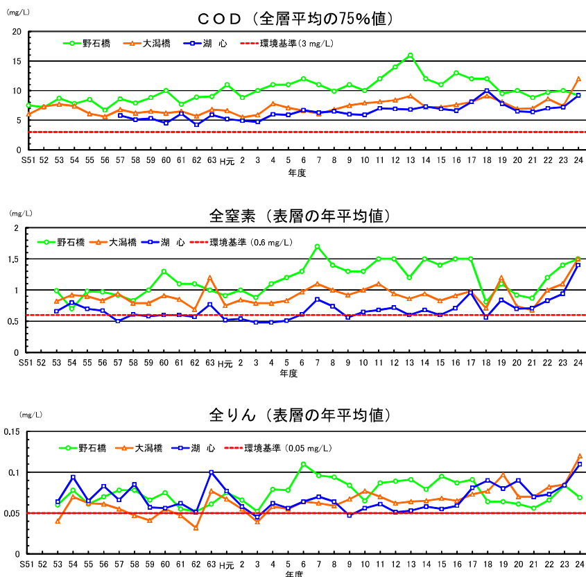
八郎湖の水質の経年変化
